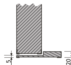
Bundstykke Type 3
